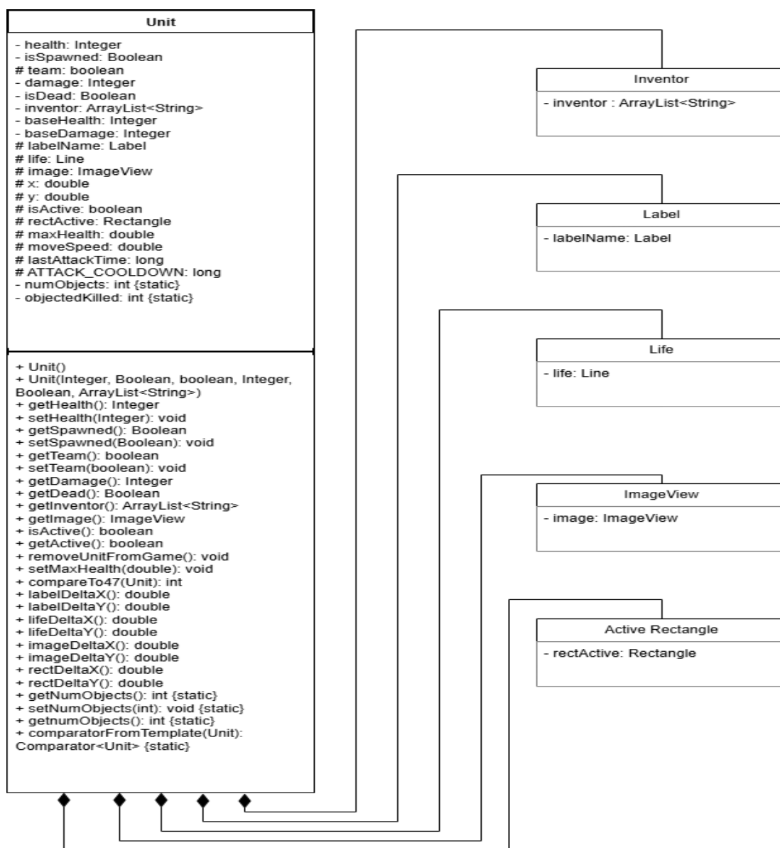
Рисунок 3.3 – Діаграма композиції
