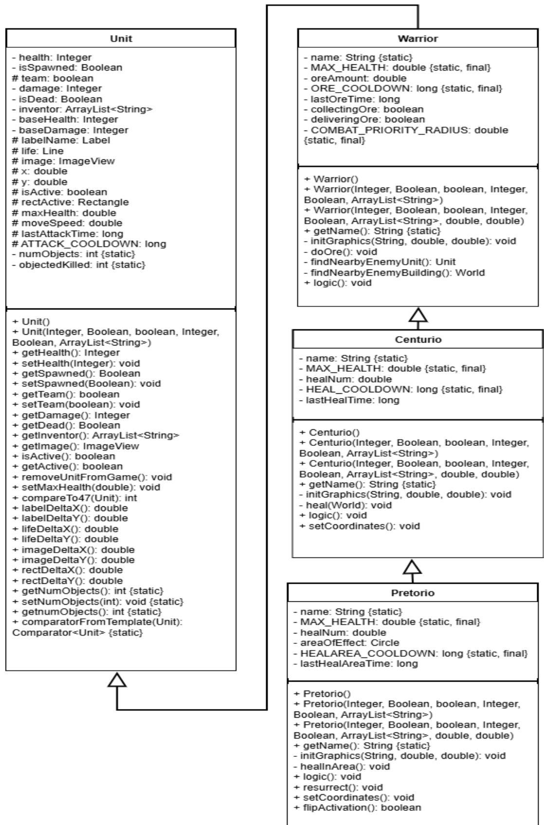
Рисунок 3.1 – Діаграма наслідування
